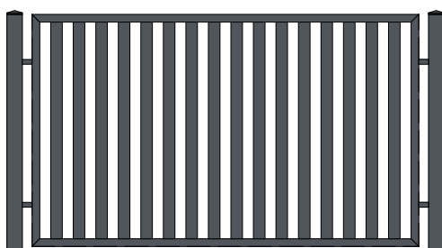
profil zamknięty 60x20 prześwity pomiędzy profilami 50-60mm
