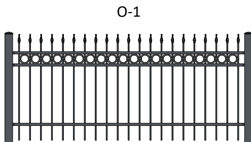
pręt pełny 12x12 prześwity pomiędzy prętami 100mm
