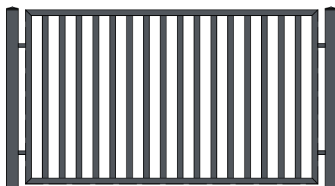
profil zamknięty 40x20 prześwity pomiędzy profilami 60-80mm
