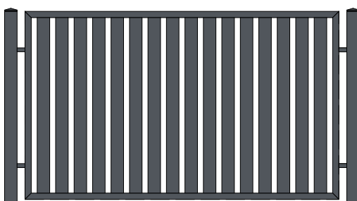
profil zamknięty 80x20 prześwity pomiędzy profilami 30-40mm
