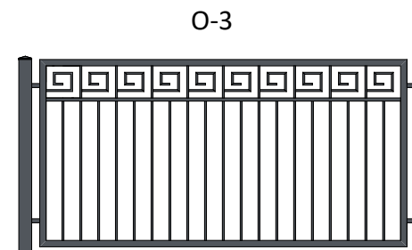
pręt pełny 12x12 prześwity pomiędzy prętami 100mm
